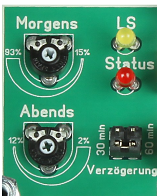
Abbildung 1: Einstellpaneel HK
