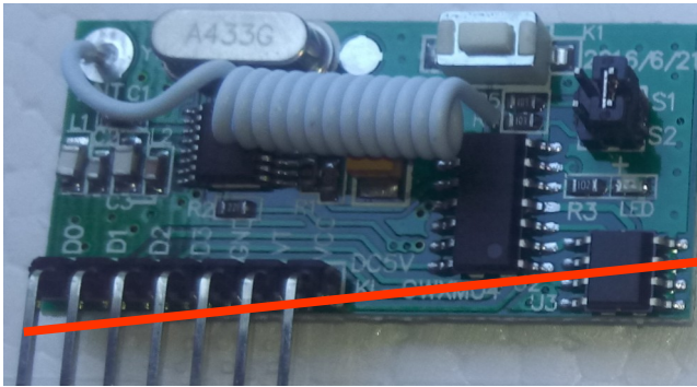
Abbildung 4: Funkempfänger
